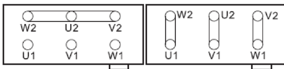
соединение «звезда»
