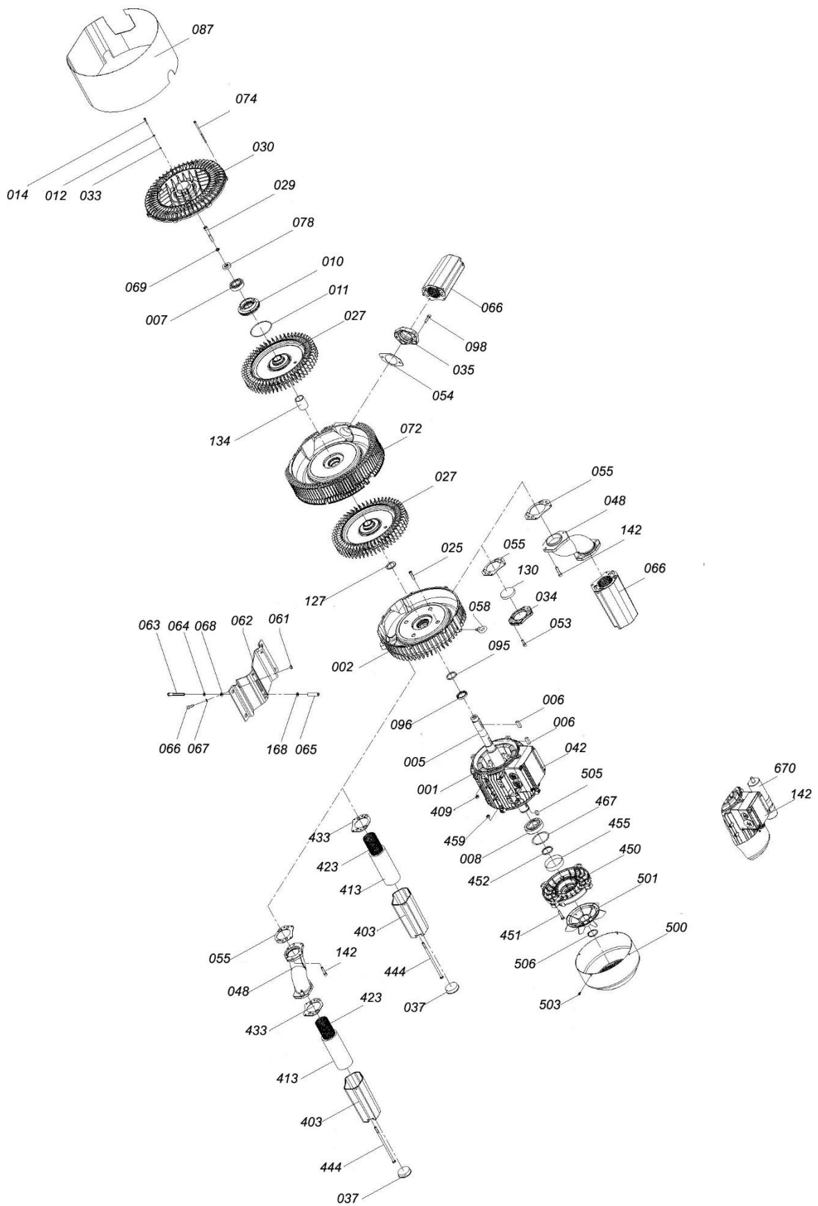
Рис. 3 – Детализовка двухступенчатых воздуховок 2RB
