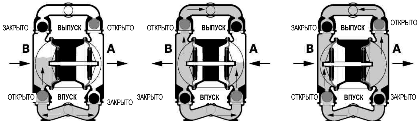
РИС. 1 клапан направляет сжатый воздух на заднюю часть диафрагмы А. Сжатый воздух подается непосредственно жидкостную камеру, разделенную эластомерными диафрагмами. Диафрагма действует как разительная мембрана между сжатым воздухом и жидкостью, уравнивает нагрузку и снимает механическое напряжение с диафрагмы. Сжатый воздух удаляет диафрагму от центра насоса. Другая диафрагма натягивается валом, соединенным с диафрагмой под давлением. Диафрагма В находится на стороне всасывания; воздух за диафрагмой выпускается в атмосферу через выпускное отверстие насоса. Движение диафрагмы В по направлению к центру насоса создает вакуум в камере В. Атмосферное давление перемещает жидкость во входной коллектор, а шарик всасывающего клапана смещается. Жидкость может теперь перемещаться через шарик всасывающего клапана и заполняет жидкостную камеру (см. затемненную область).
