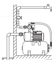
Fig. 2 Работа выше уровня жидкости
