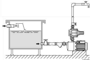
Fig. 1 Работа под гидравлическим напором
