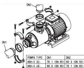
Fig. 8 Порты Victaulic
